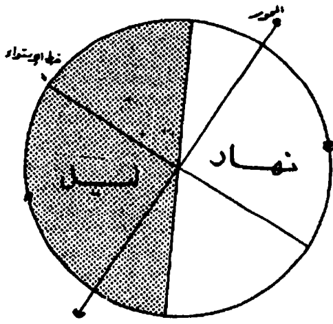
حدوث الليل والنهار نتيجة لكروية الأرض
